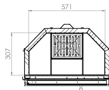
PRZEKRÓJ A-A
