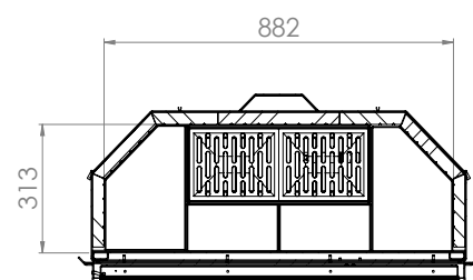
PRZĘKRÓJ A-A
